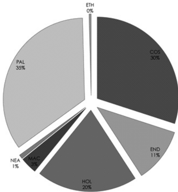
Figure 2. Biogeographic origin of Azorean freshwater invertebrates. Percentages of each origin are shown. PAL-Palaearctic; ETH-Ethiopian; COS-Cosmopolitan; END-Endemic; HOL-Holarctic; MAC-Macaronesian; NEA-Nearctic. Origen biogeográfico de los invertebrados acuáticos de Las Azores. Porcentajes para cada región biogeográfica considerada. PAL-Paleártico; ETH-Etíope; COS-Cosmopolita; END-Endémico; HOL-Holártico; MAC-Macaronésica; NEA-Neártica.
