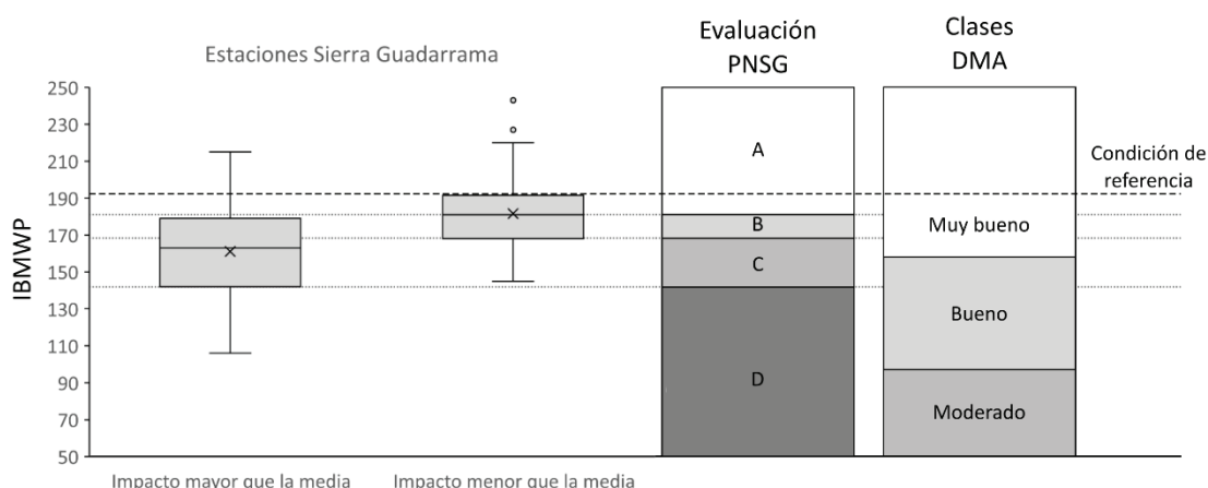
Figura 6. Distribución de los valores del IBMWP en las estaciones con impactos acumulados por encima o por debajo de la media observada en la Sierra de Guadarrama: media, mediana, cuartiles, máximo, mínimo y puntos anómalos. A la derecha se muestran los intervalos correspondientes tanto a las clases de la DMA (R-T11), como al sistema de evaluación y seguimiento del Parque Nacional de la Sierra de Guadarrama (PNSG). Distribution of the IBMWP values in the stations with cumulative impacts above or below the average observed in the Sierra de Guadarrama: mean, median, quartiles, maximum, minimum and anomalous points. On the right are the intervals corresponding to the WFD (R-T11) classes and also the evaluation and monitoring system of the Sierra de Guadarrama National Park (PNSG).
