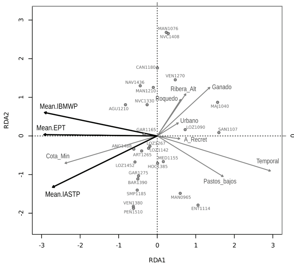
Figura 5. Análisis de redundancia (RDA), triplot con los índices biológicos (negro), las características de cuenca más relevantes e impactos (gris), y las estaciones de muestreo (gris claro). Redundancy analysis (RDA), triplot with the biological indices (black), the most relevant basin characteristics and impacts (grey), and the sampling stations (light grey).
