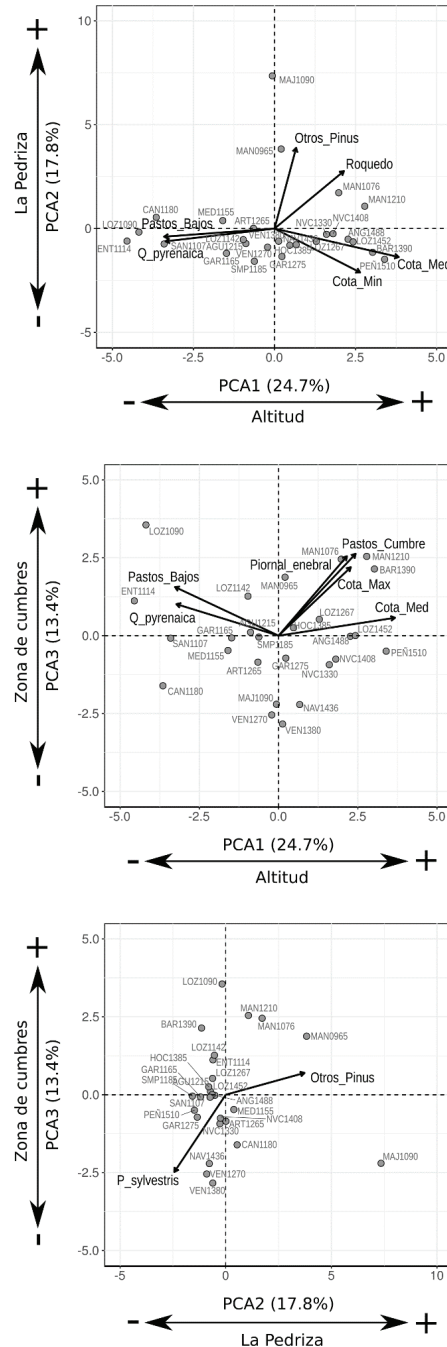
Figura 4. PCA biplot mostrando el primer, segundo y tercer componente con las variables morfométricas de la cuenca y los diferentes tipos de vegetación (sólo se han representado las variables con Cos^2 > 0.6 ). Los puntos son las distintas estaciones de muestreo. PCA biplot showing the first, second and third components with the morphometric variables of the catchment and the different vegetation typologies (only the variables with Cos^2 > 0.6 have been represented). Points are the different sampling stations.
