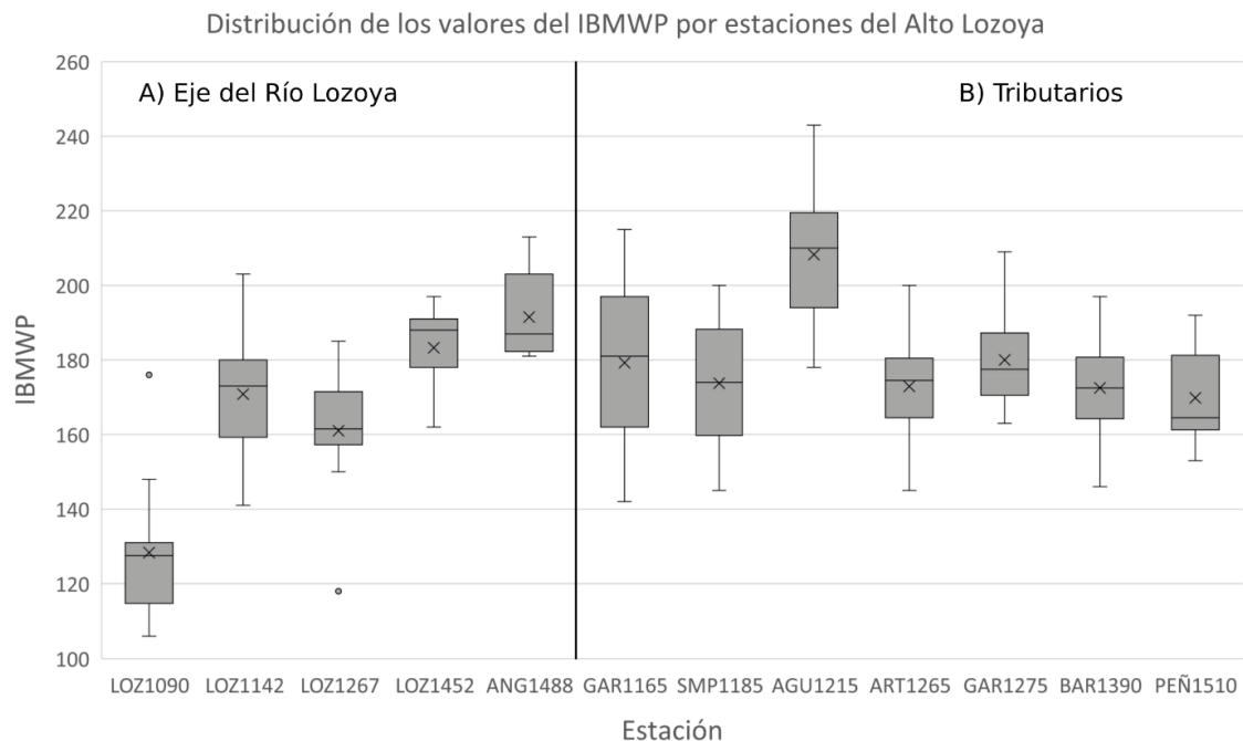
Figura 2. Distribución de los valores del IBMWP por estación de muestreo en los cursos fluviales permanentes: media, mediana, cuartiles, máximo, mínimo y puntos anómalos. A) estaciones del eje del río Lozoya. B) estaciones situadas en tributarios. Ordenadas de izquierda a derecha por altitud en ambos casos. Distribution of the IBMWP values by sampling station in the permanent streams: mean, median, quartiles, maximum, minimum and anomalous points. A) stations on the axis of the Lozoya River. B) stations located in tributaries. Ordered from left to right by altitude in both cases.
