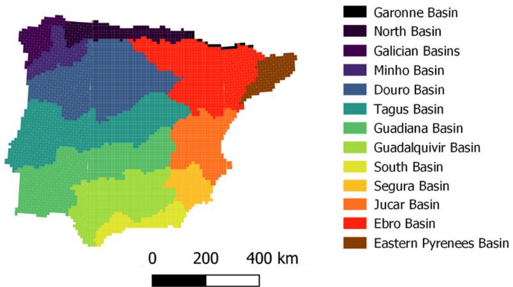
Figure S1. Map of the Iberian basins. Mapa de las cuencas ibéricas.
